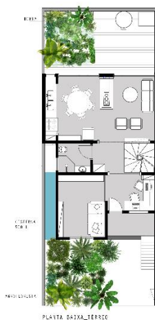
Fig. 2 Planta do pavimento térreo.
